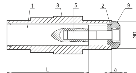
MONTAGE / MONTAJE
