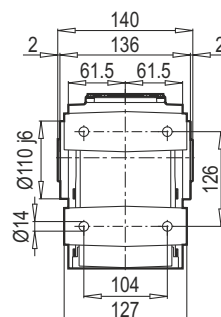
DA / B14
