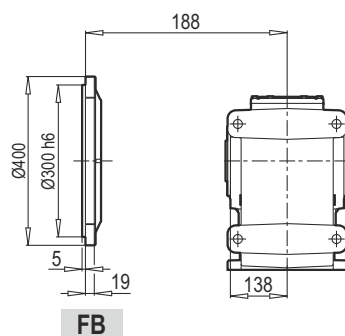
DG / B5
