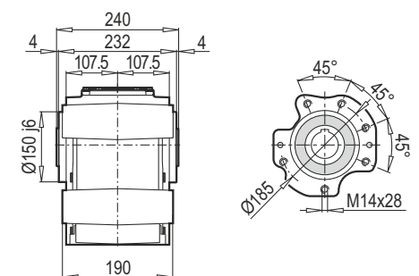
DG / B14
