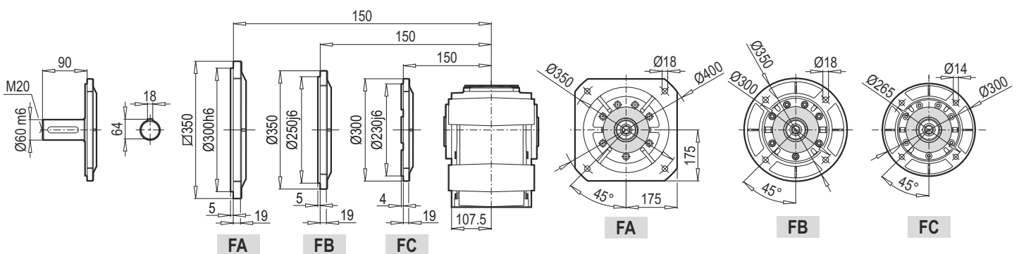
DG / B5
