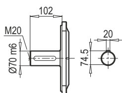
TMG / B5
